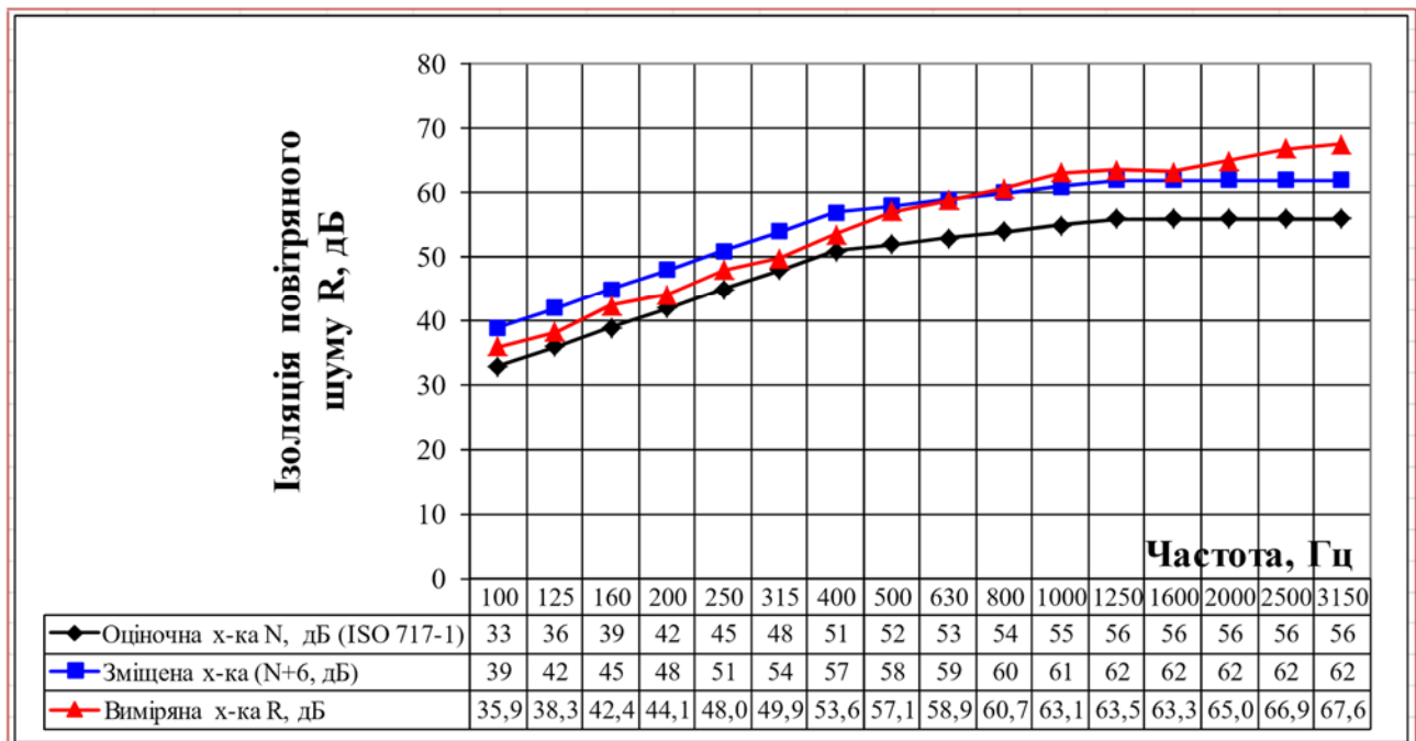
Рисунок 3 – Частотна характеристика ізоляції повітряного шуму ( R , дБ) зовнішньої стіни товщиною 200 мм із газобетонних блоків густиною 600 кг/м 3 із фасадним вентиляльованим утепленням системи «СКАНРОК»
