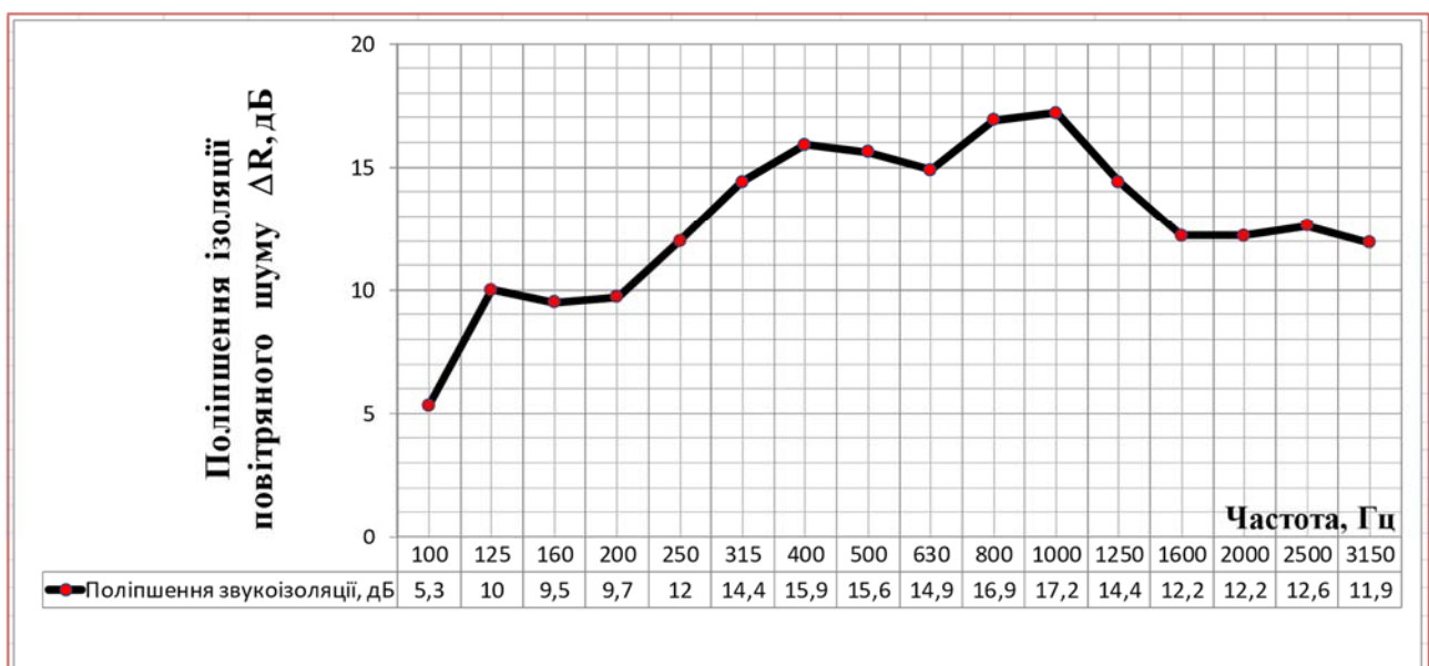
Рисунок 4 – Частотна характеристика поліпшення ізоляції повітряного шуму ( \Delta R , дБ) зовнішньої стіни товщиною 200 мм із газобетонних блоків густиною 600 кг/м 3 за рахунок улаштування системи утеплення «СКАНРОК»
