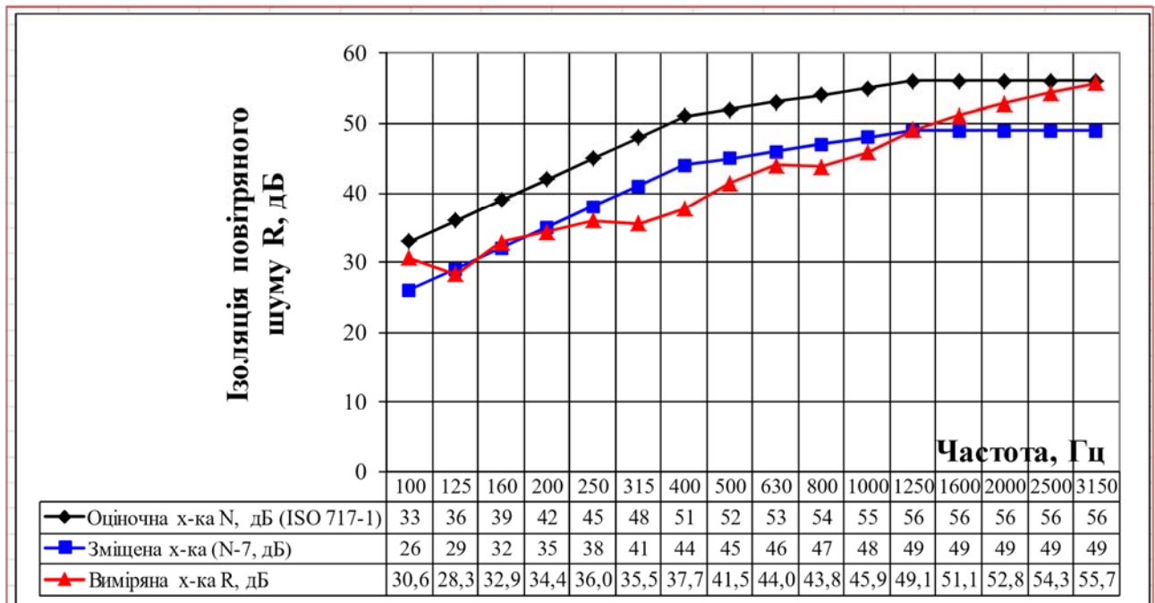
Рисунок 2 – Частотна характеристика ізоляції повітряного шуму ( R , дБ) зовнішньої стіни товщиною 200 мм із газобетонних блоків густиною 600 кг/м 3 (без системи утеплення)
